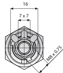
Koniec cylindra
