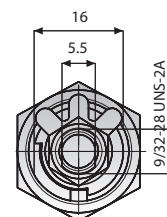
Koniec cylindra
